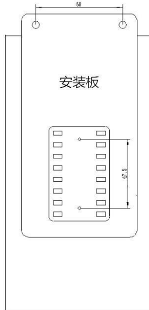
安装板安装
