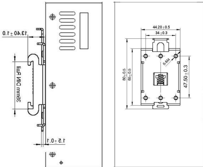
导轨式安装
